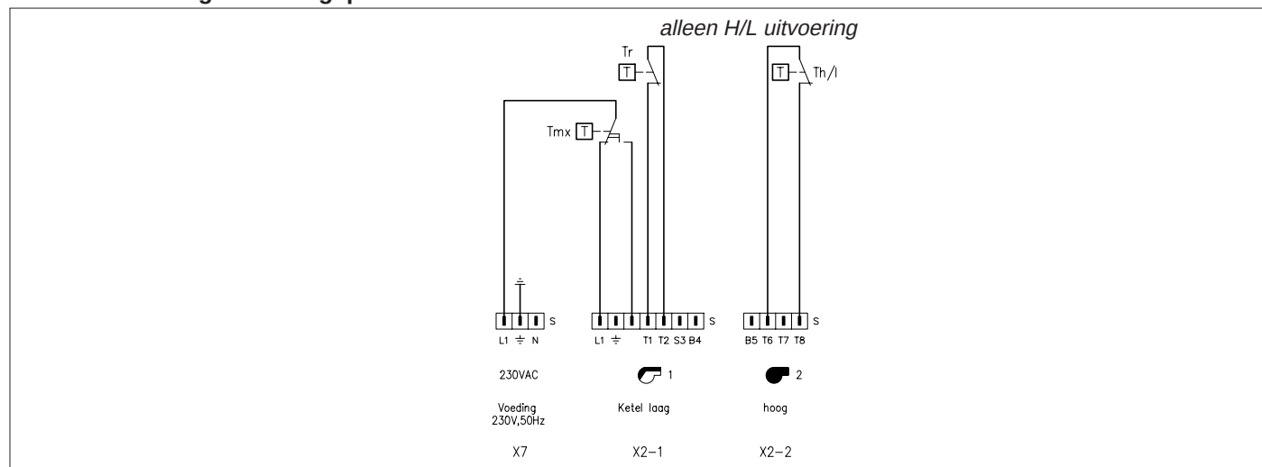
Afb. 06 Eenvoudig bedieningspaneel
