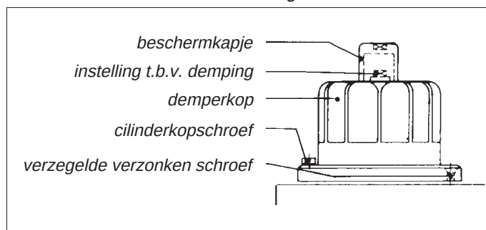
Afb. 13 Demperkop beveiligingsafsluiter
