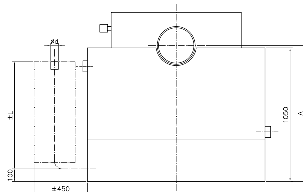
bovenaanzicht
