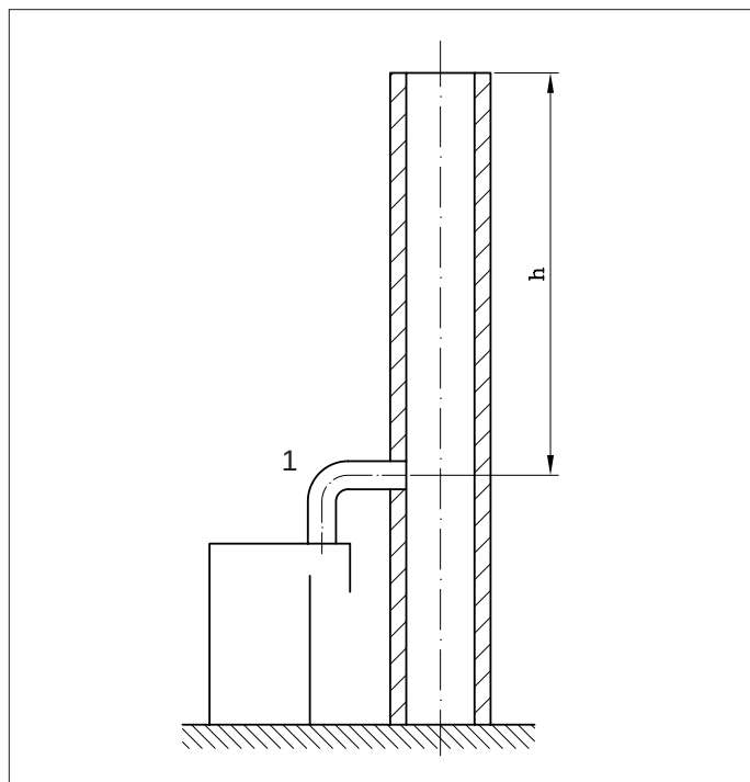
Afb. 02 Verbrandingsgasafvoersysteem
