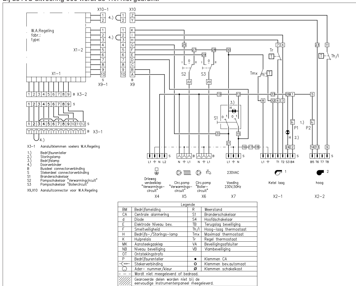
Afb. 07 Uitgebreid bedieningspaneel
