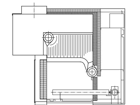
doorsnede
