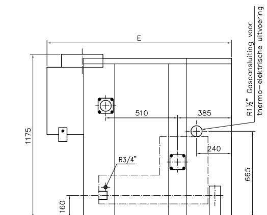
linkerzijaanzicht
