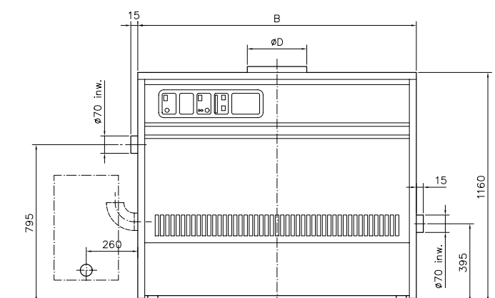
vooraanzicht
