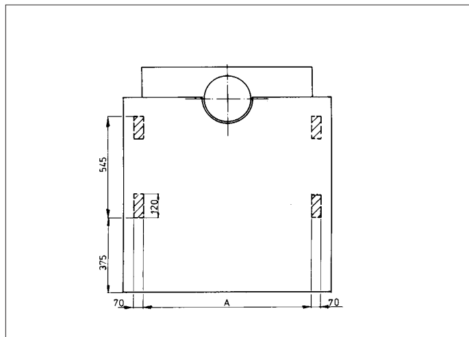
Afb. 04 Steunoppervlak
